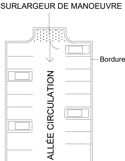
Figure 5-23 Surlargeur de manœuvre
