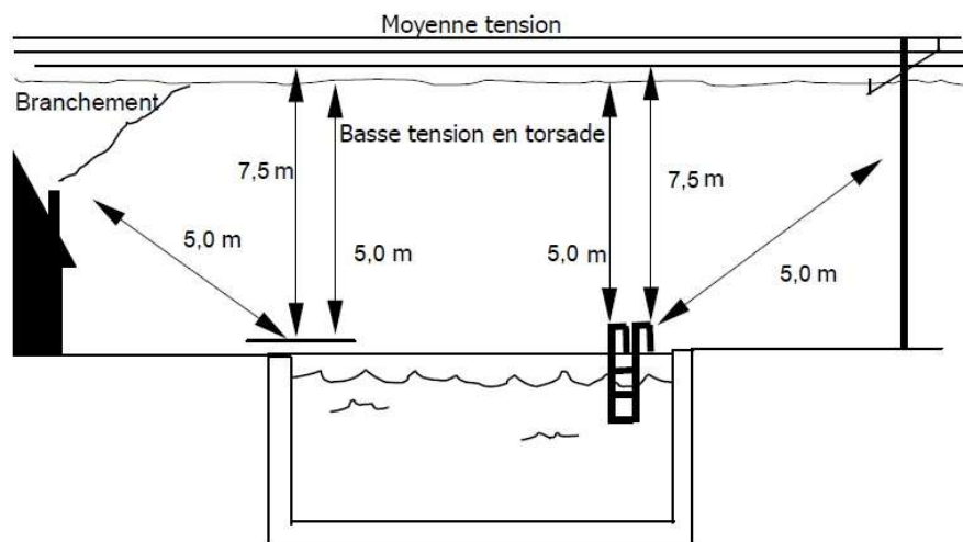
Figure 7-33 Implantation d'une piscine creusée en fonction du réseau électrique aérien
