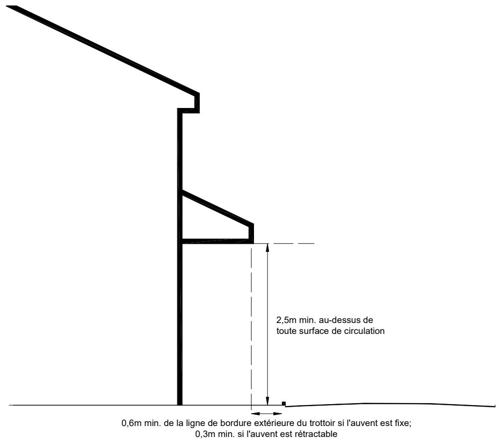
Figure 10-41 Distance minimale entre la projection au sol de l'auvent et la limite de terrain avant et la hauteur libre sous l'auvent
