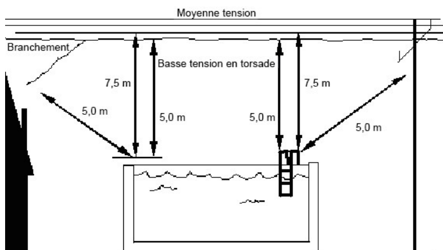
Figure 5-19 Implantation d'une piscine hors terre en fonction du réseau électrique aérien
